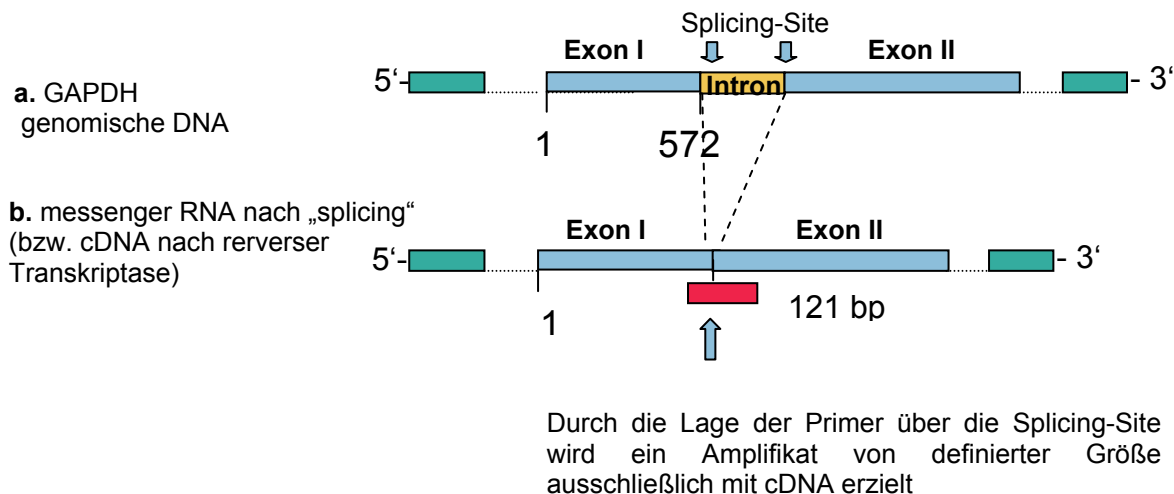
Abbildung 3: Diskriminierung genomischer DNA von cDNA durch Lage der Primer über eine Splicing-Site. Bei der genomischen DNA erfolgt keine Primerbindung im Bereich des Introns (a). Durch die Positionierung des forward Primers über die splicing site kann eine Vervielfältigung in der PCR nur bei der umgeschriebenen messenger RNA (cDNA) erfolgen (b).
